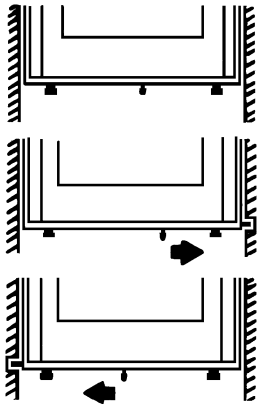
Schemi: funzionamento della barra anti-rullio
