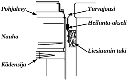
Normaaliasento, turvakiinnitys käytössä
