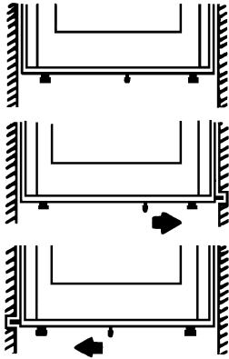
Kuvat: keinumisen estävän tangon toiminta.
