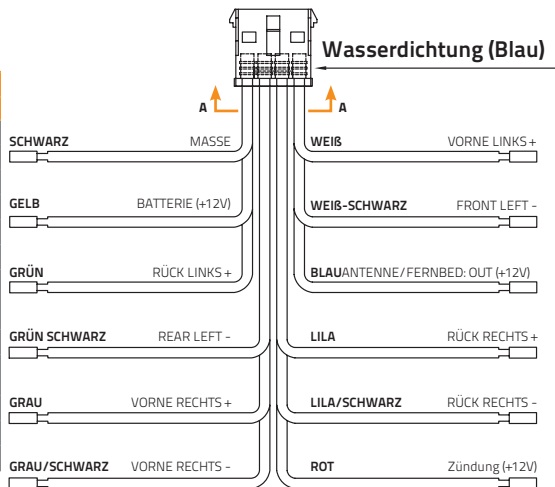
12 POLIGER KABELBAUM
