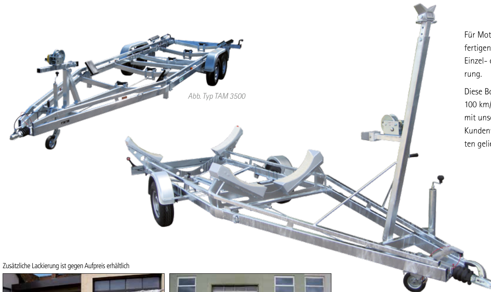
Abb. Spezialtrailer Bavaria B/one
