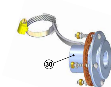
Rumpfdurchführung 2467
