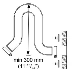
Svanhals
