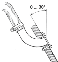
Svanhals
