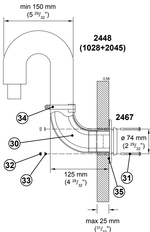
Rumpfdurchführung 2467 instal- liert. Die Einbauöffnung hat einen Durchmesser von \varnothing 50 mm und die Einschraublöcher sind 4 x \varnothing 6 mm
