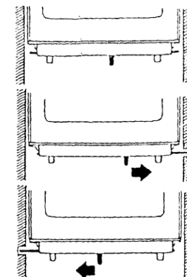
Schemor: krängningshämmarens funktion
