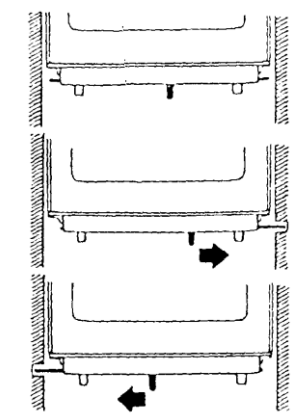
Schemi: funzionamento della barra anti-rullio
